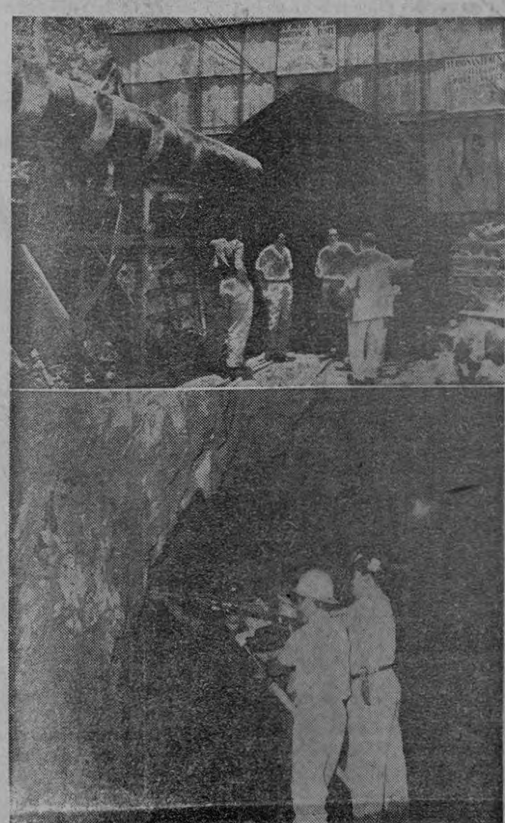
Esta es la entrada del túnel al pie del Cerro de La Marina, en el valle de Oroquieta. Cuadrilla de barreteros trabajando a 385 metros de profundidad, en el Proyecto N° 1 del Río Macho
